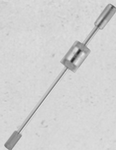
Klz. kladivo pre vnút. vyťahovač ložísk Obj.č. 0714 525 030
