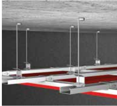
Zarážacia hmoždinka W-ED/S Obj.č. 0904 010 ...
